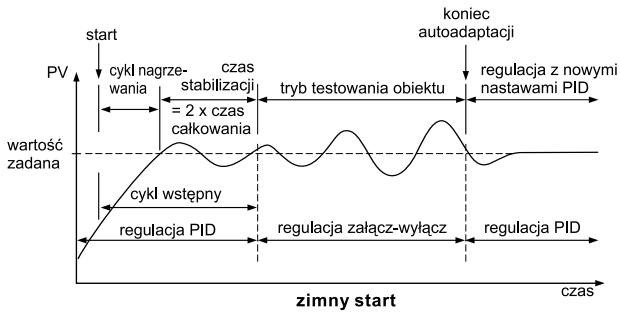
Rys. 62. Autoadaptacja dla zimnego startu.
