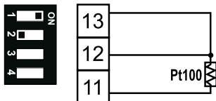
linia 3-przewodowa
