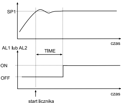
Rys.43. Funkcja timera czasu wyrzewnania.
