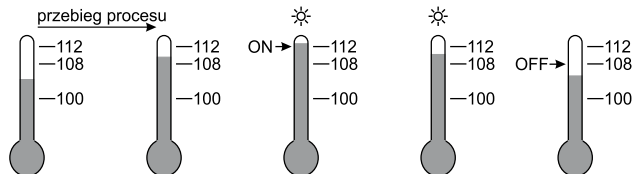
Rys.48. Alarm względny normalny.
