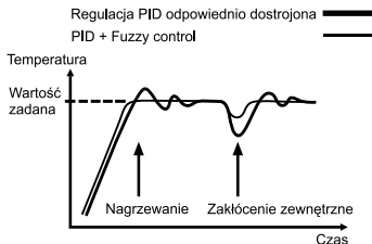
Rys.1. Korzyści z zastosowania funkcji fuzzy-logic.
