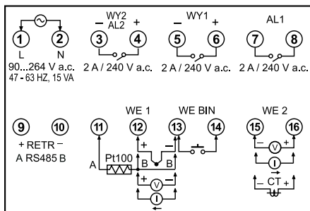
Rys. 9. Opis listwy zaciskowej.
