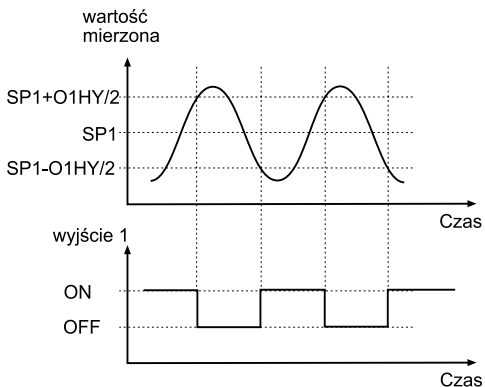
Rys.41. Regulacja załącz-wyłącz typu grzanie
