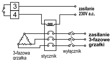
Rys.27. Wyjście typu przełącznik lub triak do sterowania stycznikiem trójfazowym
