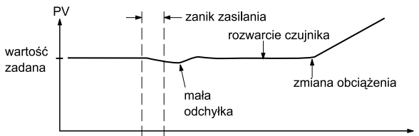
Rys.61. Praca regulatora w trybie awaryjnym z przełączeniem bezuderzeniowym.
