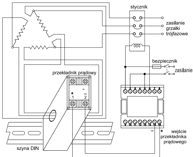
Rys. 18. Podłączenie przekładnika prądowego do grzałki trójfazowej
