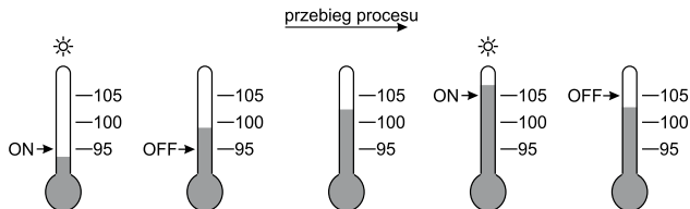
Rys.52. Alarm względny zewnętrzny normalny.
