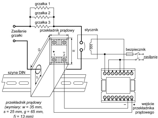
Rys. 17. Podłączenie przekładnika prądowego do grzałki jednofazowej
