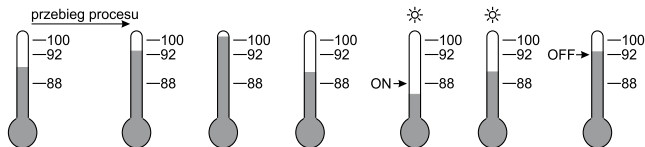
Rys.50. Alarm względny z wstrzymaniem.
