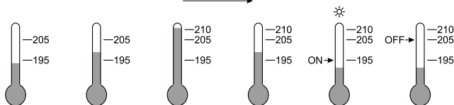
Rys.46. Alarm bezwzględny z wstrzymaniem.
