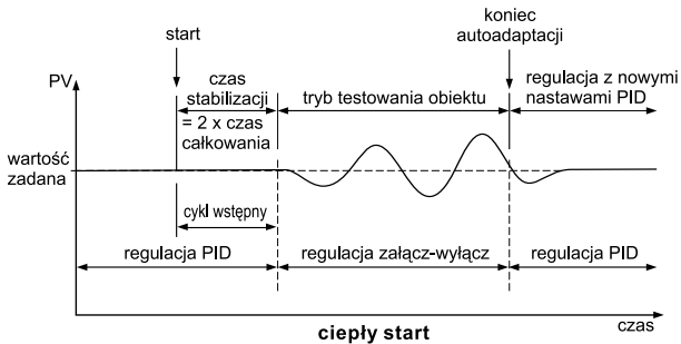
Rys. 63. Autoadaptacja dla ciepłego startu.
