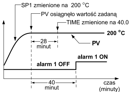
Rys.69. Timer czasu wygrzewania.
