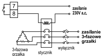
Rys.33. Wyjście typu przekaźnik do sterowania stycznikiem trójfazowym
