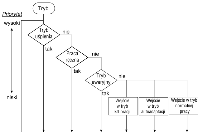
Rys. 6. Priorytet trybów pracy.
