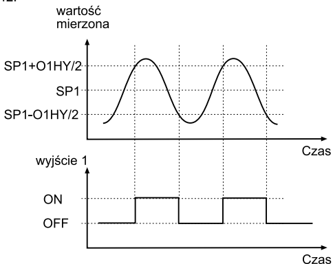
Rys.42. Regulacja załącz-wyłącz typu chłodzenie
