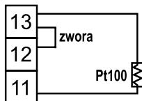
linia 2-przewodowa
