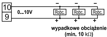
Rys.38. Wyjście retransmisyjne napięciowe
