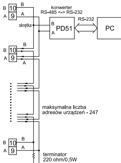
Rys.36. Podłączenie RS-485
