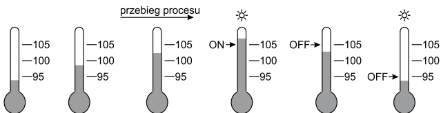
Rys.54. Alarm względny zewnętrzny z wstrzymaniem.
